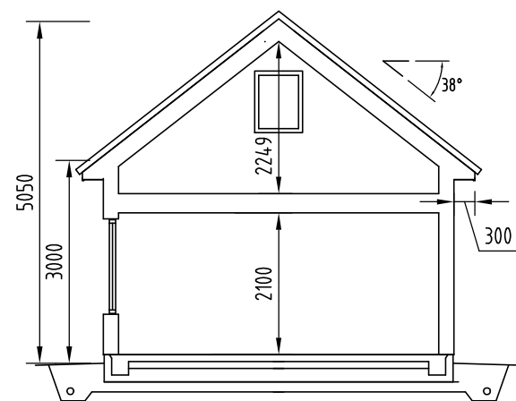
SEKTION A-A
