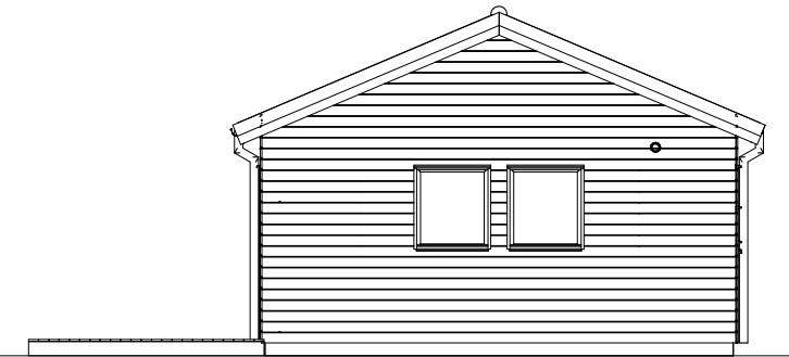
FASAD B
