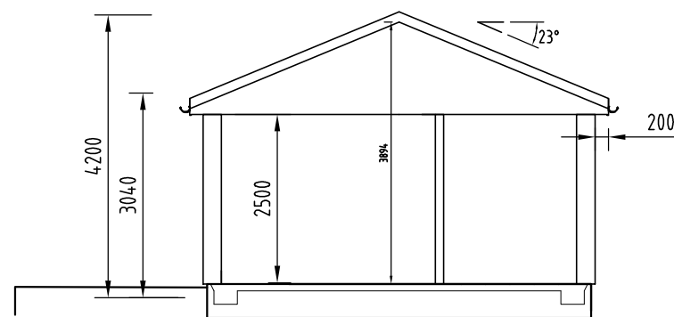
SEKTION A-A
