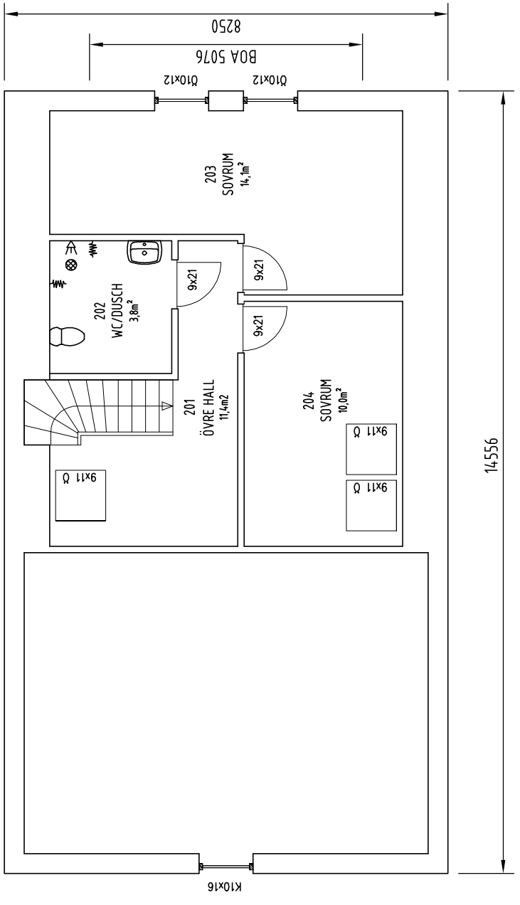
ÖVRE PLAN Boyta 39,3 m 2
